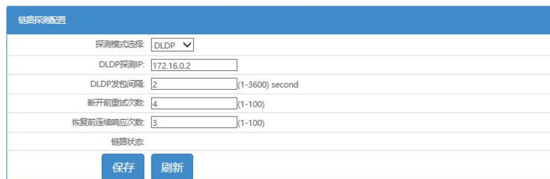
图 4-20 DLDP 配置界面
