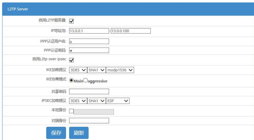
图 4-35 L2TP 服务端配置
